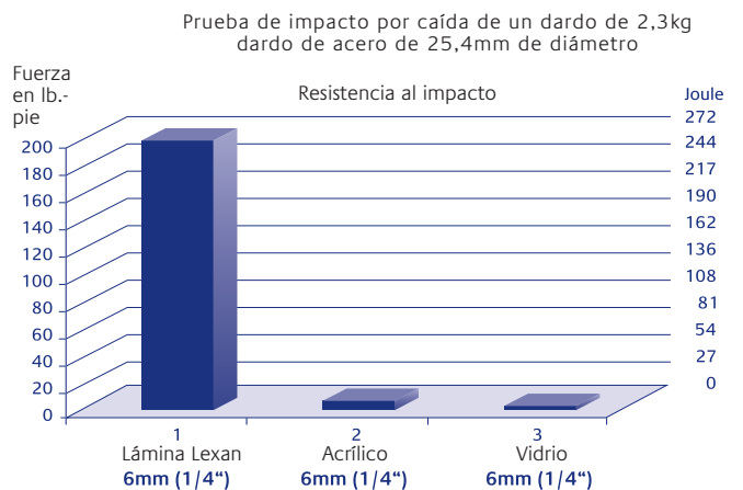
Figura 1 Resistencia a los impactos
