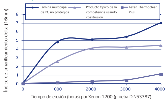
Figura 3 Índices de amarillamiento (iA) por la exposición a la intemperie
